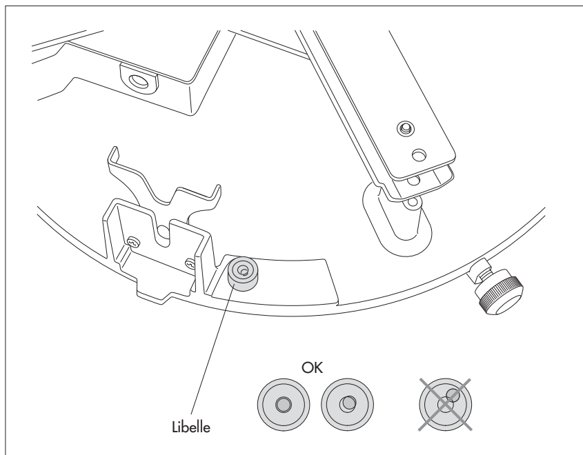
Abb. 15: Ausrichten des OTT Pluvio 2 L.
