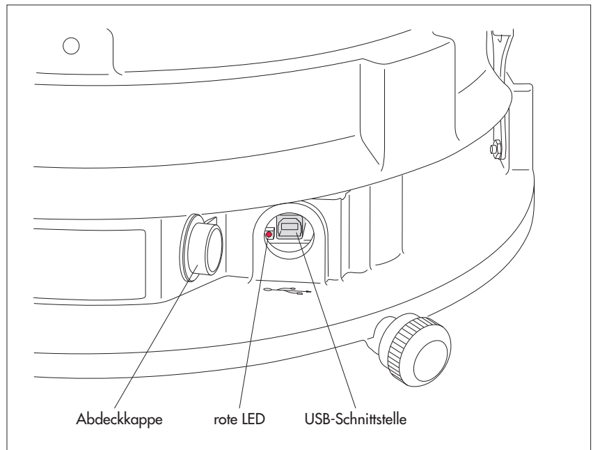
Abb. 18: Funktionskontrolle durchführen.
