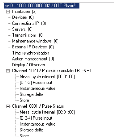
Abb. A7: Beispielkonfiguration eines OTT netDL mit 2 aufgezeichneten Messwerten.
