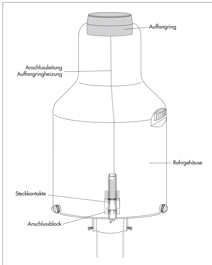
Abb. 4: Prinzipdarstellung der OTT Pluvio 2 L Auffangringheizung.
