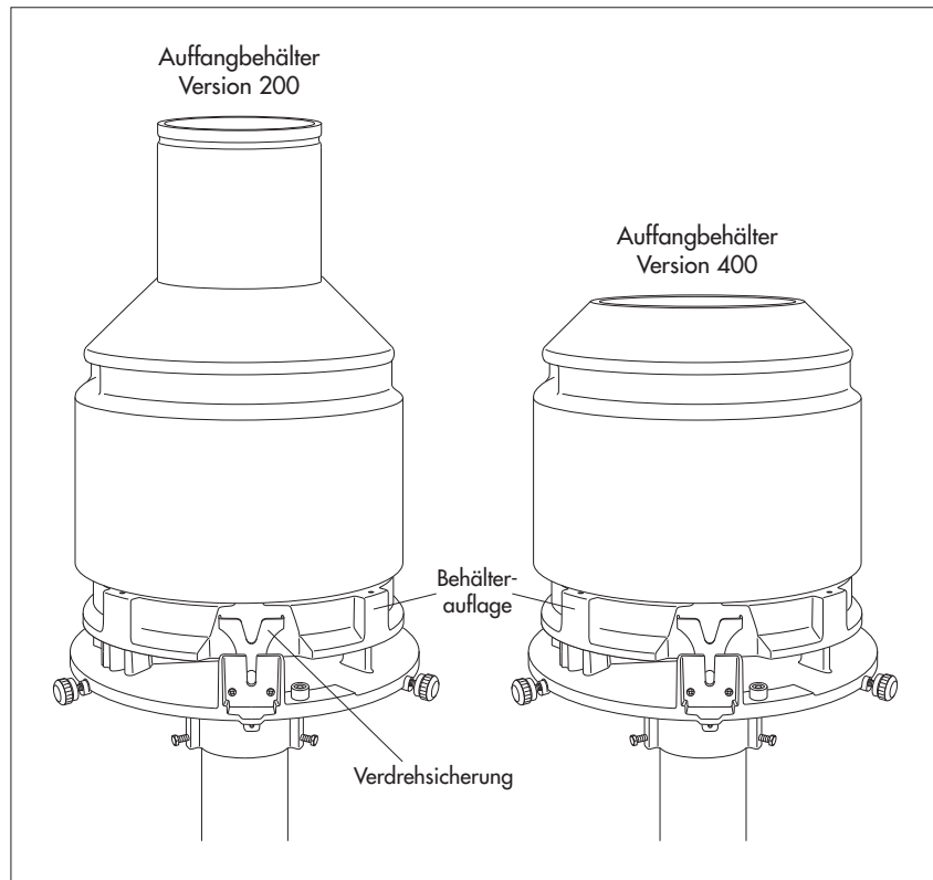
Abb. 17: Auffangbehälter auf Behälterauflage aufsetzen.
