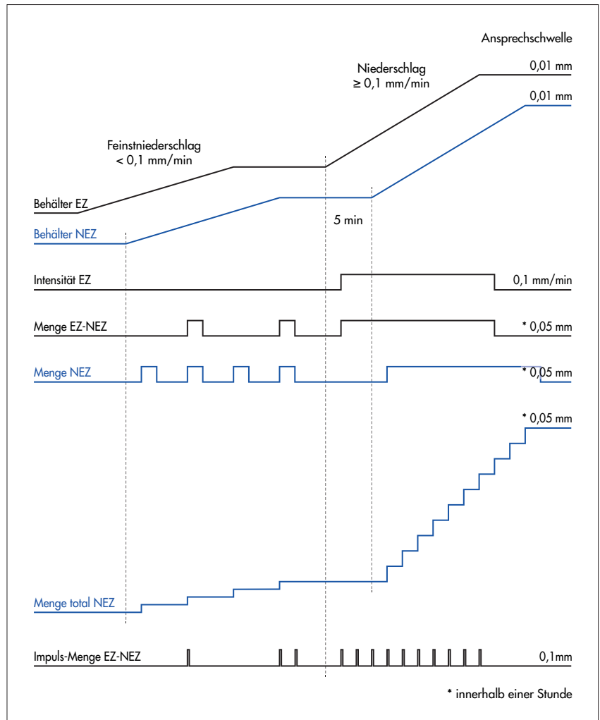
Abb. 3: Schematische Darstellung der Ausgabe der verschiedenen Niederschlagsmesswerte des OTT Pluvio 2 L für Feinstniederschlag (< 0,1 mm/min) und Niederschlag (≥ 0,1 mm/min).
