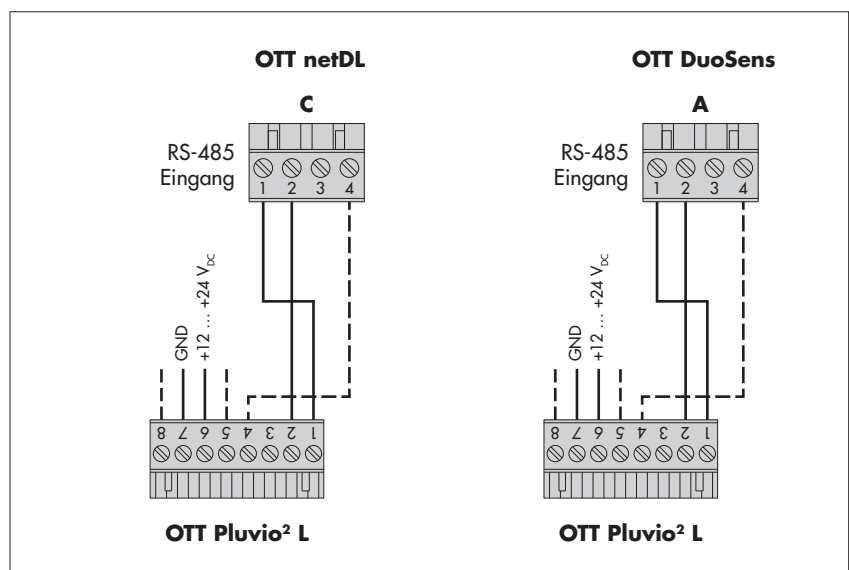
Abb. A2: OTT Pluvio 2 L über RS-485-Schnittstelle (SDI-12-Protokoll) an OTT netDL oder OTT DuoSens anschließen.
