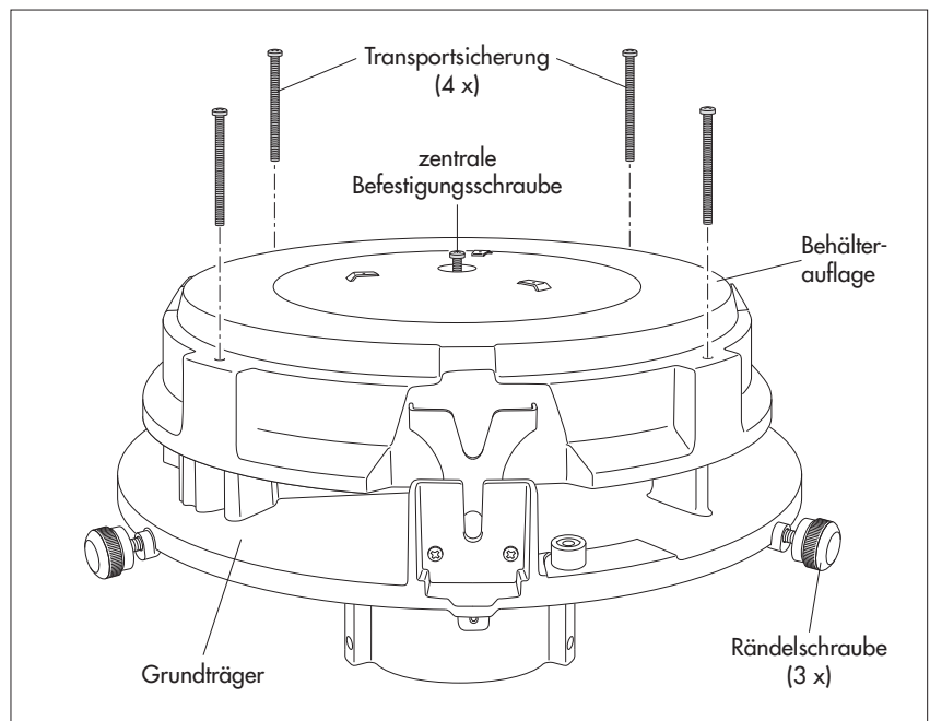
Abb. 8: Transportsicherung entfernen und Behälterauflage abnehmen.
