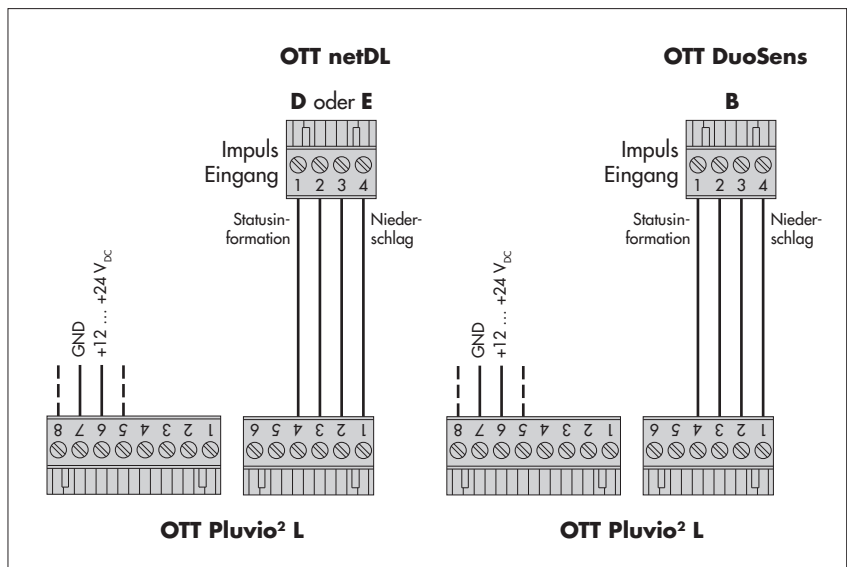
Abb. A5: OTT Pluvio 2 L über Impulsausgang an OTT netDL oder OTT DuoSens anschließen.
