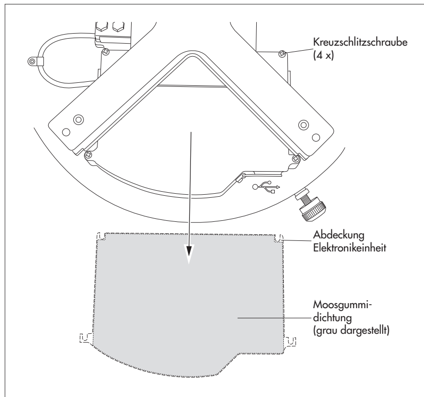
Abb. 9: Abdeckung der Elektronikeinheit abnehmen.
