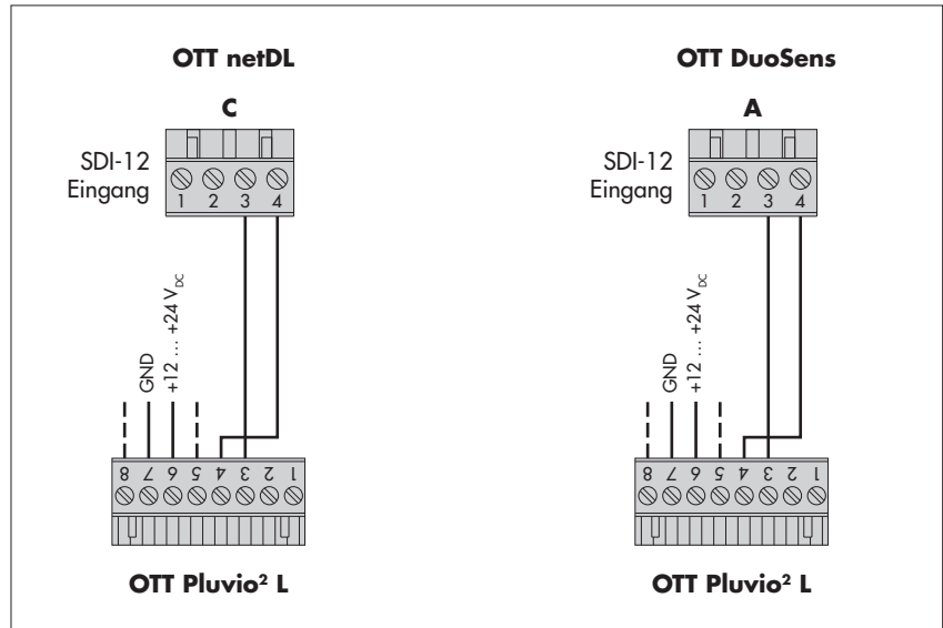
Abb. A1: OTT Pluvio 2 L über SDI-12-Schnittstelle an OTT netDL oder OTT DuoSens anschließen.
