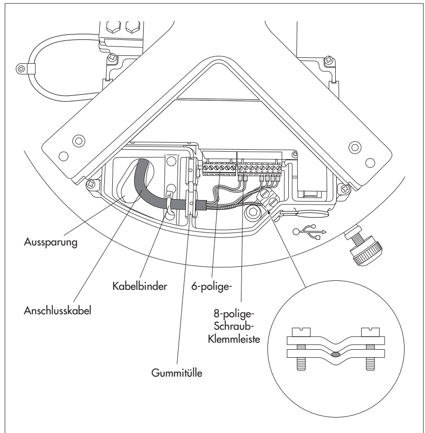
Abb. 13: Anschlusskabel in der Elektronikeinheit kontaktieren.
