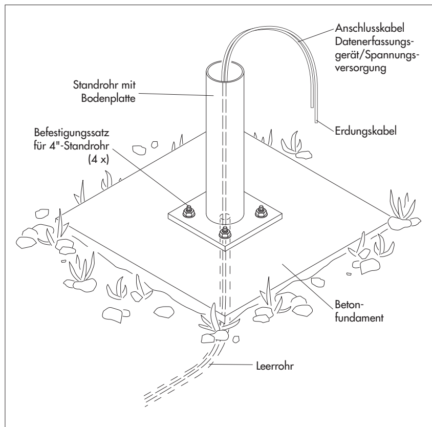
Abb. 7: Für die Installation des OTT Pluvio 2 L vorbereiteter Aufstellort.
