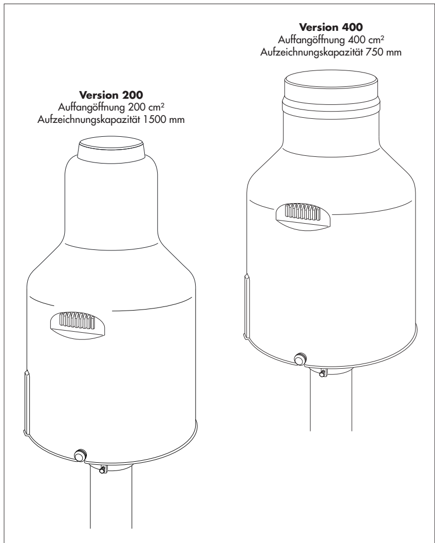
Abb. 1: Niederschlagssensor OTT Pluvio 2 L. Der OTT Pluvio 2 L ist in zwei Ausführungen lieferbar: Version 200 und Version 400.
