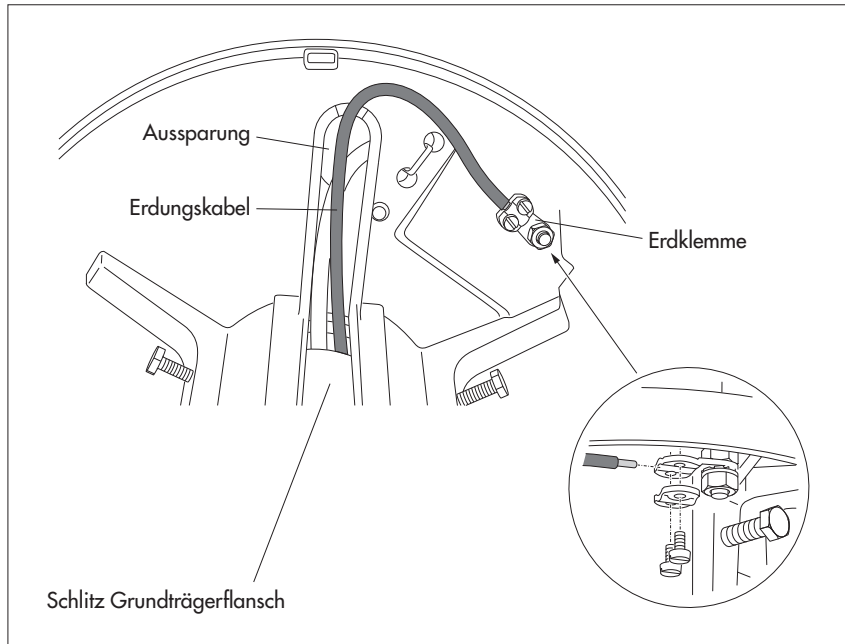
Abb. 14: Erdungskabel anschließen (Blickrichtung von unten).
