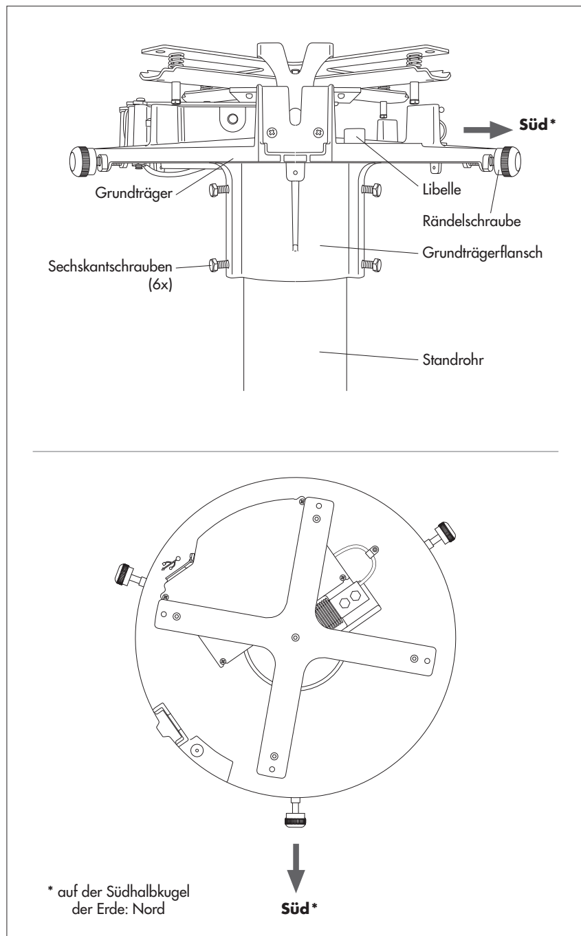
Abb. 12: Grundträger auf Standrohr installieren.
